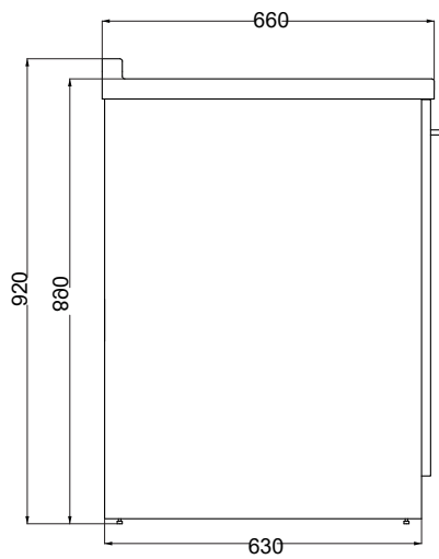
VISTA LATERALE
