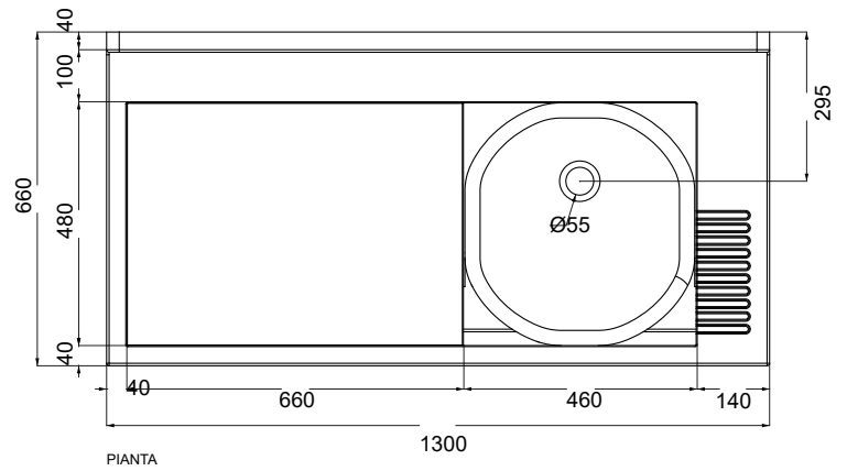
PIANTA
